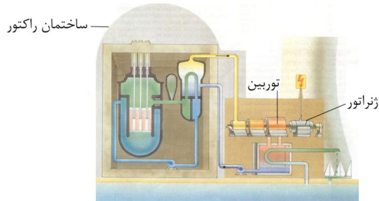
شکل ۱. فرآیند تولید برق در ساختمان‌های راکتور و توربین در یک نیروگاه هسته‌ای با آب تحت فشار
