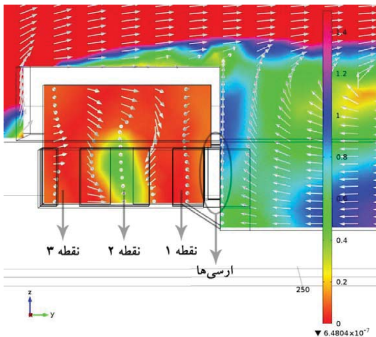
شکل ۷: برش طولی اتاق اصلی درحالی که ارسی‌ها بسته هستند.
