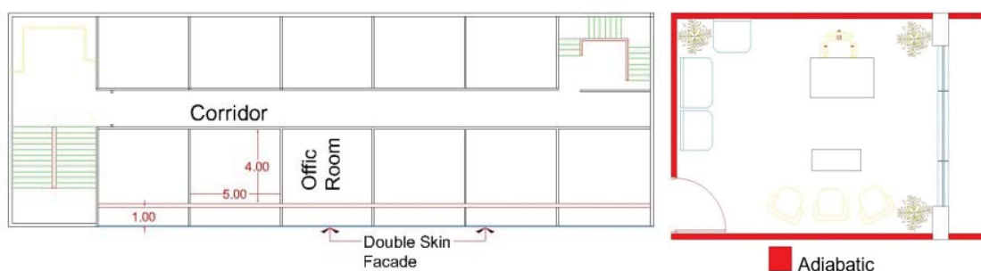
شکل ۱۰: پلان مجموعه‌ی اداری (سمت راست)؛ پلان یکی از اتاق‌های اداری به همراه نواحی آدیباتیک (سمت چپ)
