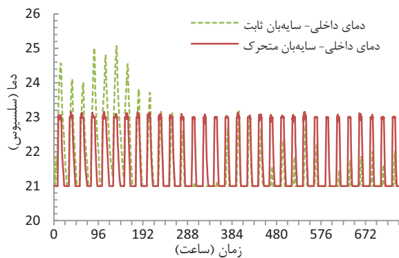
شکل ۱۵. نمودار دمای داخلی برای حالات سایه‌بان متحرک و ثابت برای ماه دسامبر
