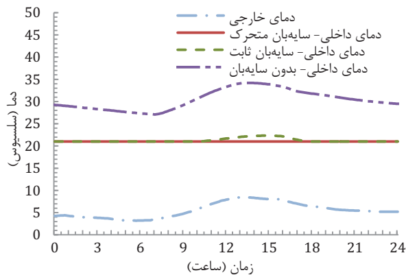
شکل ۹. نمودار دمای خارجی و دمای هوای داخلی برای سه حالت سایه‌بان متحرک، ثابت و بدون سایه‌بان برای روز ۲۲ دسامبر
