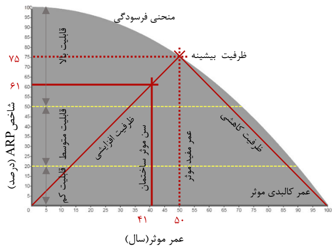
شکل ۳- مدل قابلیت استفاده مجدد انطباقی (ARP) مدرسه شهید دستغیب بندرانزلی
