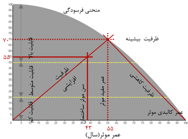
شکل ۵- مدل قابلیت استفاده مجدد انطباقی (ARP) مدرسه وحدت اسلامی بندرانزلی
