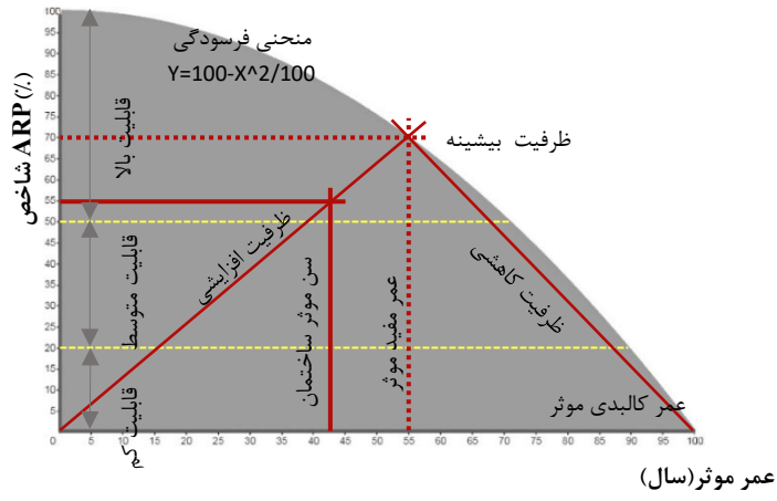
شکل ۱- مدل فرضی قابلیت استفاده مجدد انطباقی (ARP)
