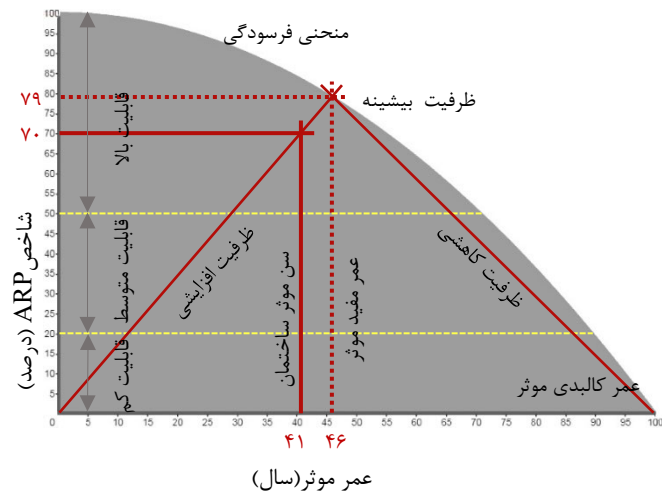
شکل ۲- مدل قابلیت استفاده مجدد انطباقی (ARP) مدرسه شهدای گمنام بندرانزلی
