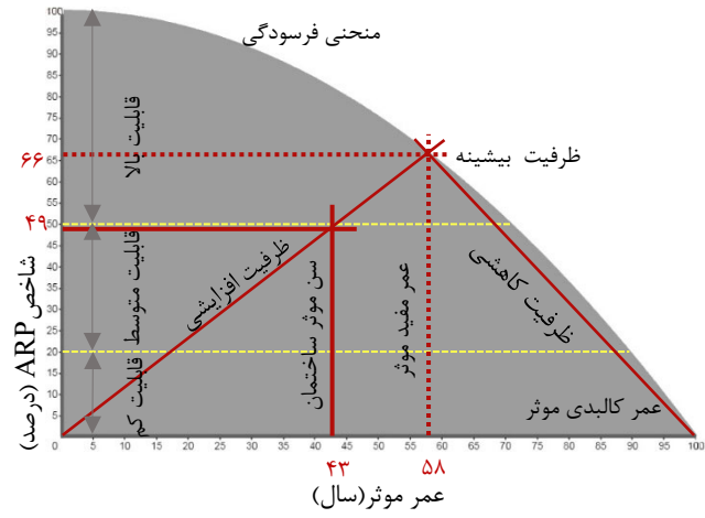
شکل ۸- مدل قابلیت استفاده مجدد انطباقی (ARP) مدرسه شهید مصطفی دوست آستانه اشرفیه
