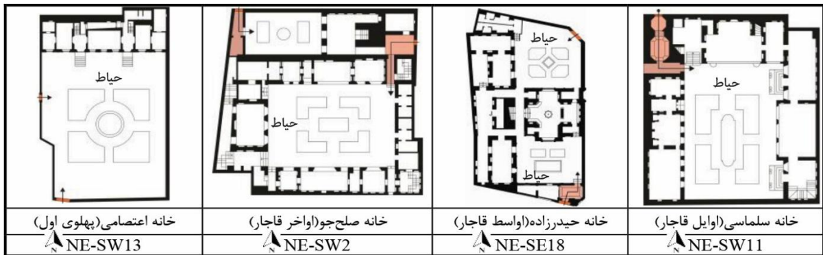
شکل ۲- محل‌گیری ورودی در نمونه‌های از خانه‌های مورد مطالعه (ماخذ: بازترسیم نگارندگان براساس (اسمعیلی سنگری و عمرانی، ۱۳۹۳))
